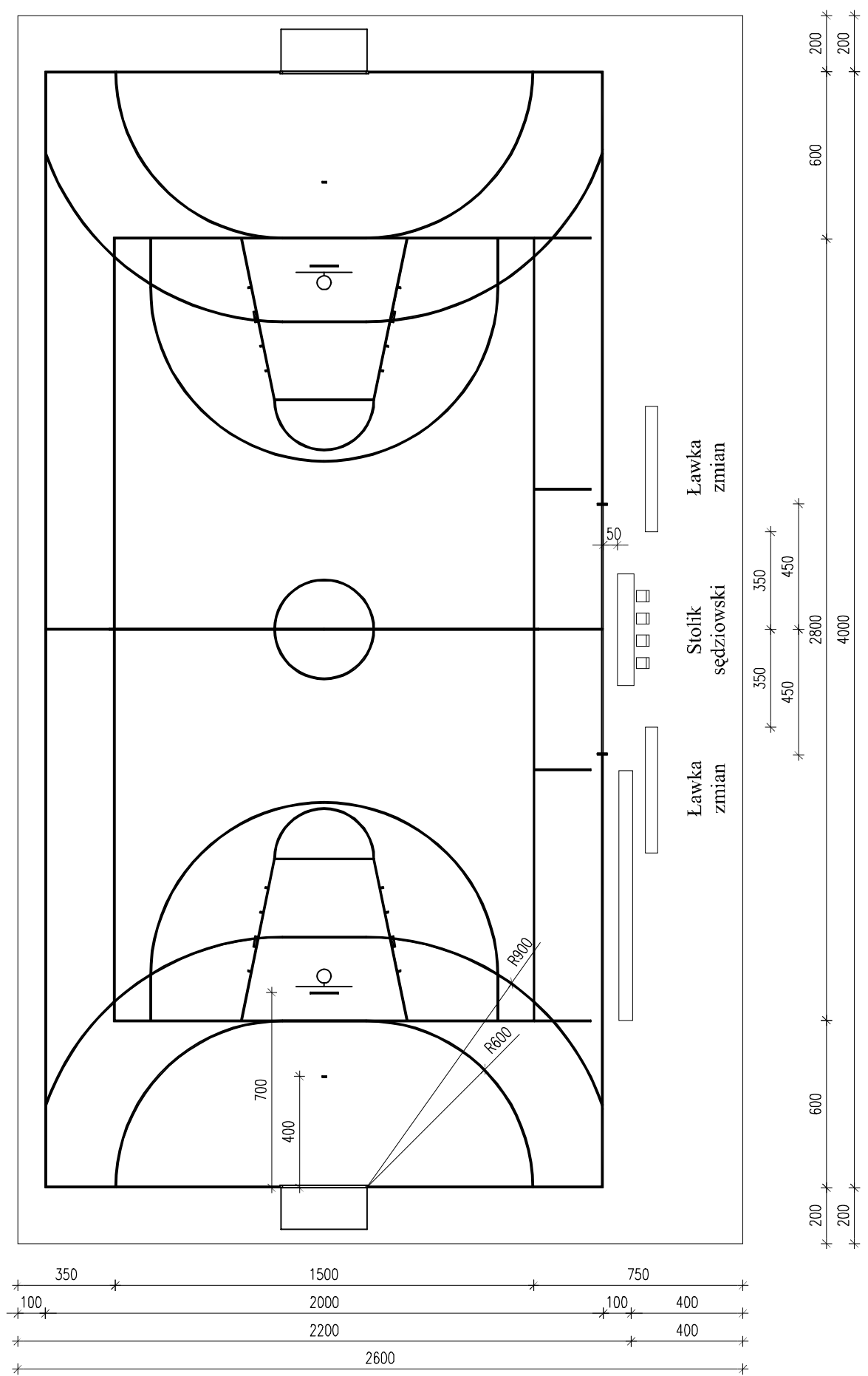
Załącznik nr 5. Schemat funkcjonalny płyty boiska hali
