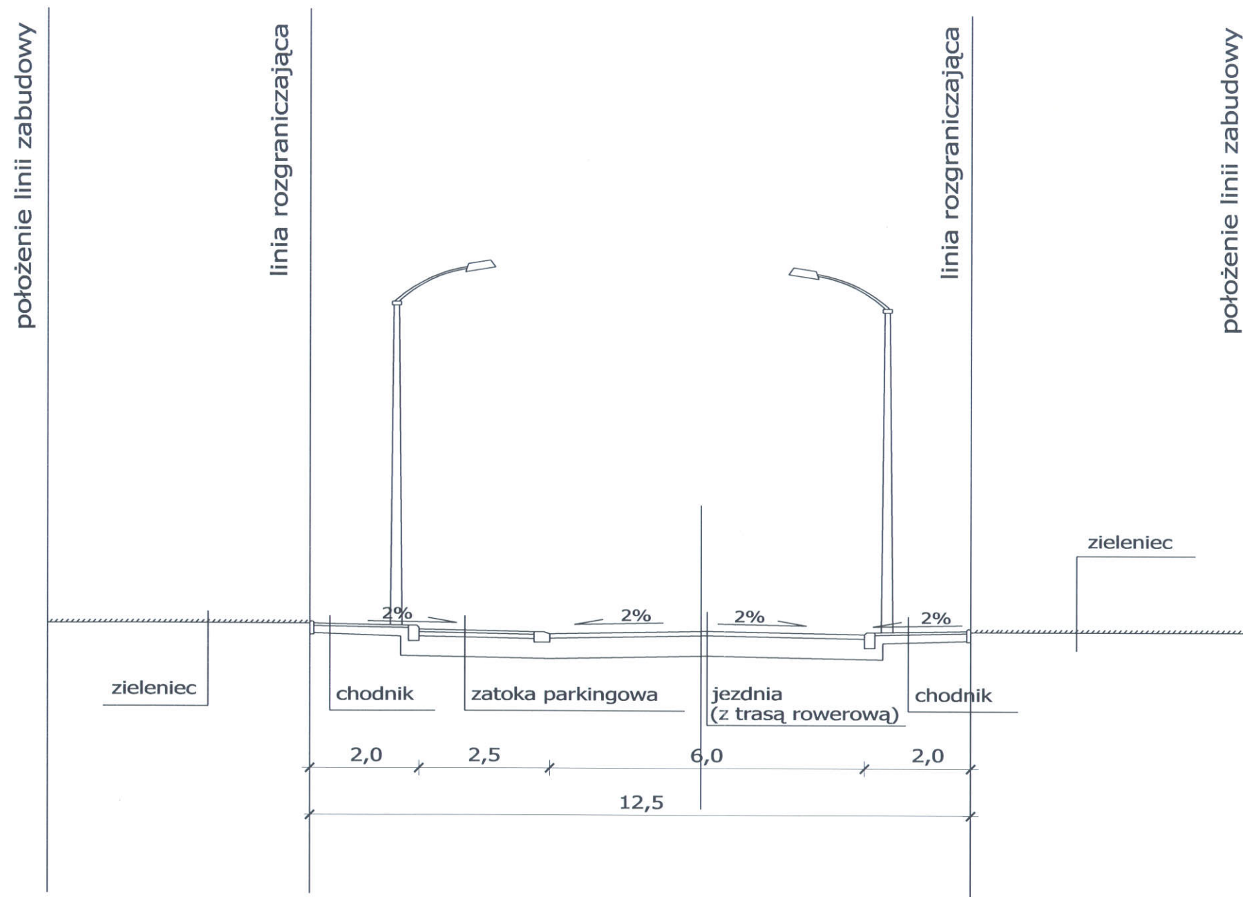
Przekrój typowy - ulica klasy KD/D (z jednostronnymi zatokami parkingowymi)
