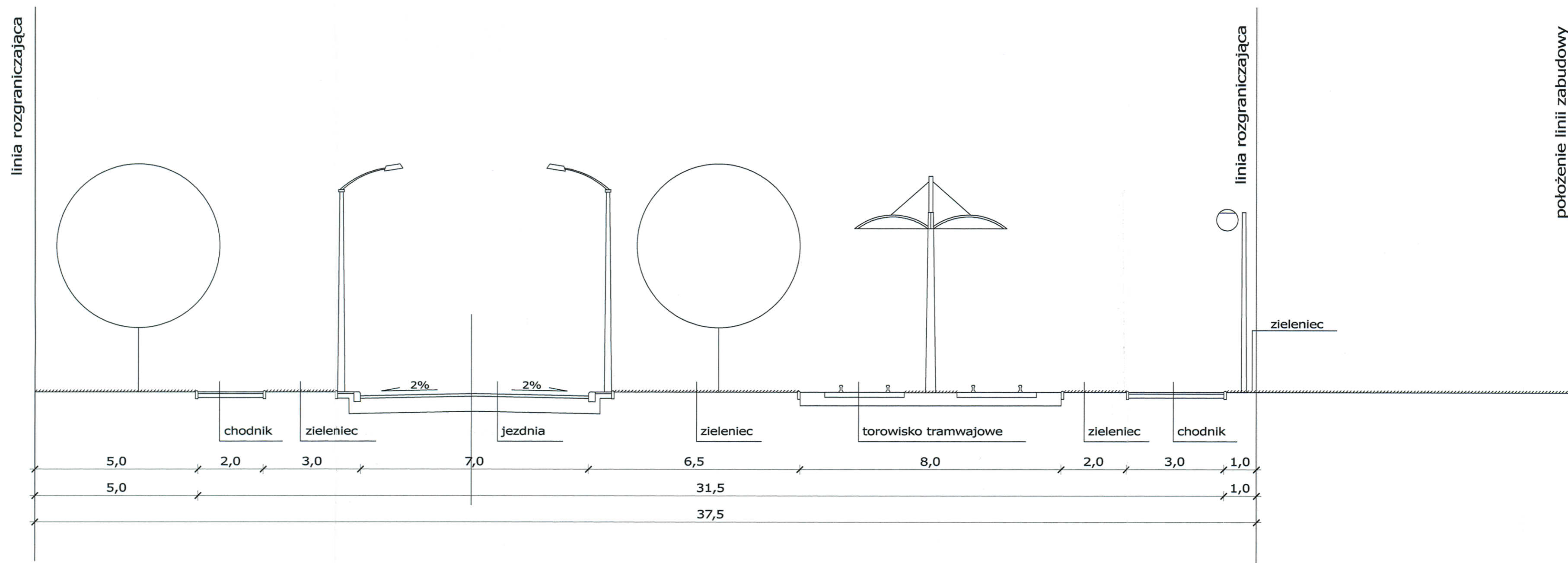
Przekrój typowy - ulica klasy KD/Z 1/2 + T
