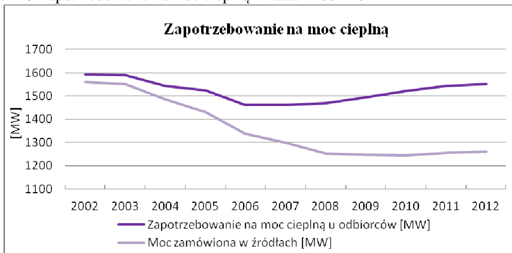
Rysunek 13 Zapotrzebowanie na moc cieplną w latach 2002-2012
